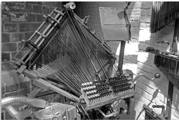
Alte Setzmaschine aus der ehemaligen Druckerei in Steyl
